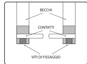
Installazione contatti
